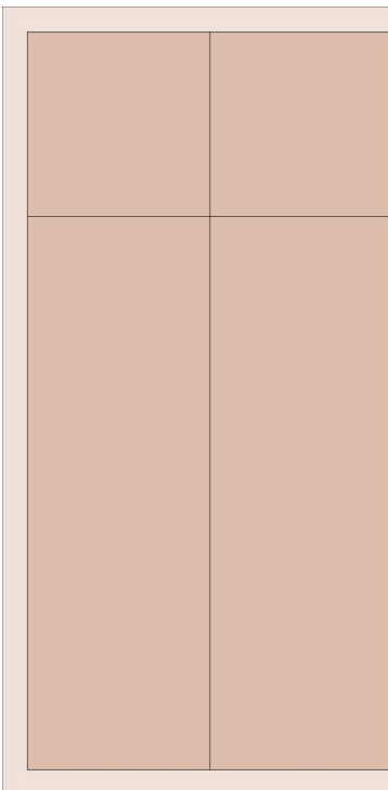
Terminale SX - BT 3 4 ante 60x60 + 60x180 LA cm. 128,3 PROF cm. 62,5 H 259,1
