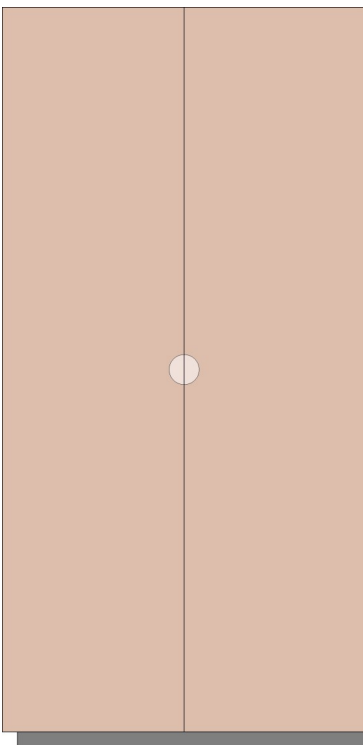
Terminale SX - BT 1 2 ante 45-60x240 LA cm. 90-120 PROF cm. 62,5 H 245
