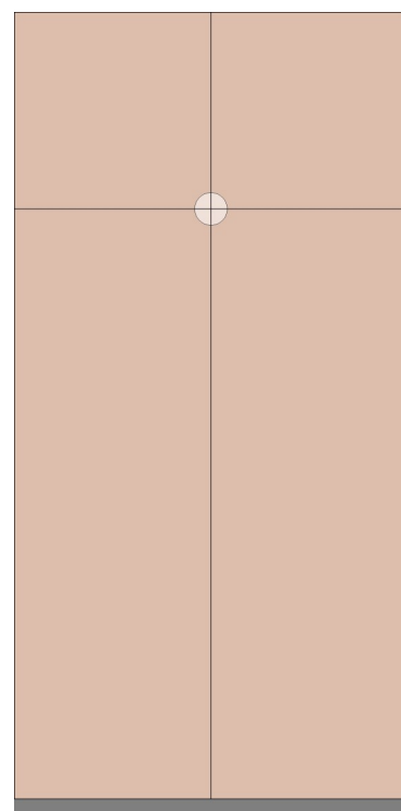
Intermedio - BE 3 4 ante 45-60x60 + 45-60x180 LA cm. 90-120 PROF cm. 62,5 H 245
